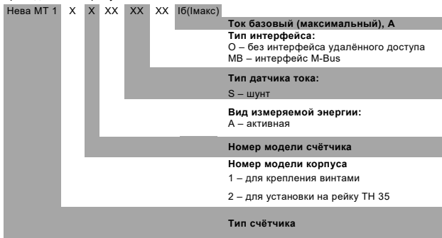
Рис. 1.1 Структура условного обозначения счётчиков НЕВА МТ 124, НЕВА МТ 112.
